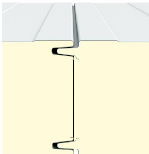
Rysunek 4.2: Przekrój płyty warstwowej IzoWall z rdzeniem poliizocyjanurowym – widoczne mocowanie
