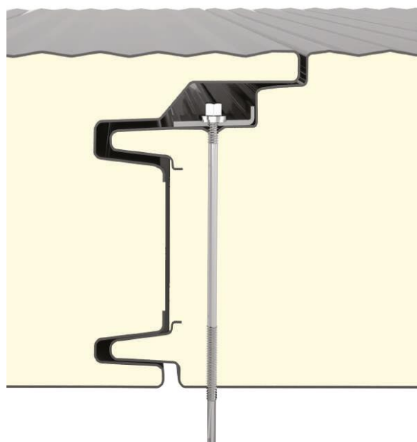
Rysunek 4.8: Przekrój płyty warstwowej IzoGold z rdzeniem poliizocyjanurowym – ukryte mocowanie
