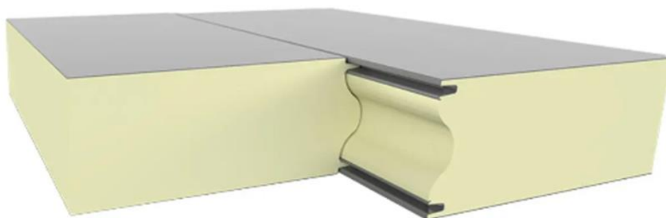
Rysunek 4.1: Płyta warstwowa IzoWall PIR-N/PIR-F
