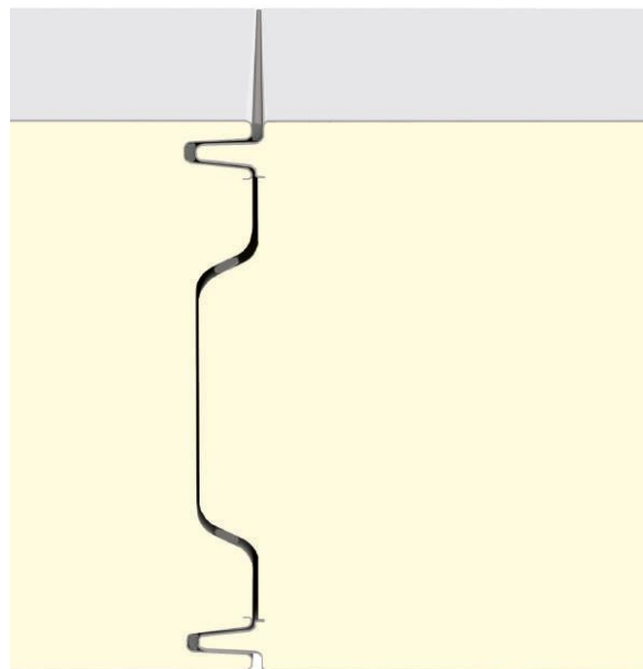
Rysunek 4.6: Przekrój płyty warstwowej IzoCold z rdzeniem poliizocyjanurowym – widoczne mocowanie
