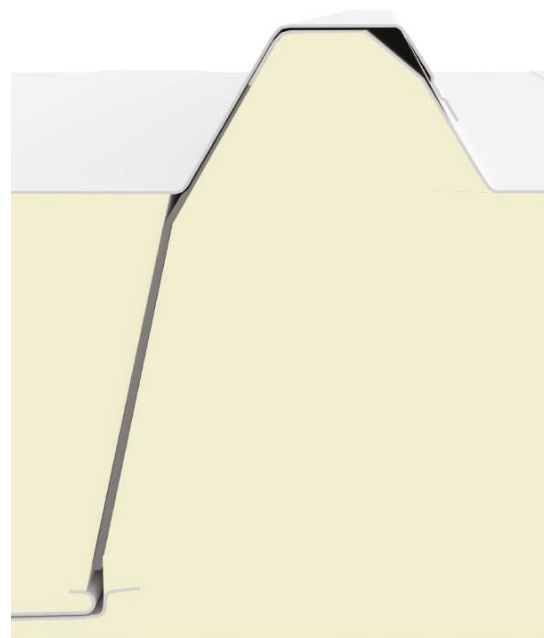
Rysunek 4.4: Przekrój płyty warstwowej IzoRoof z rdzeniem poliizocyjanurowym – wysokie profilowanie
